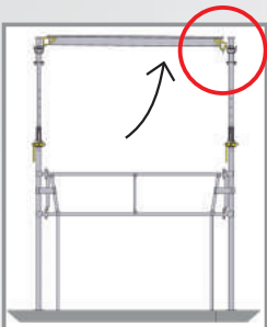
MAIOR distância entre pontaletes
