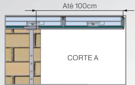
Projeção dos painéis para fora da laje
