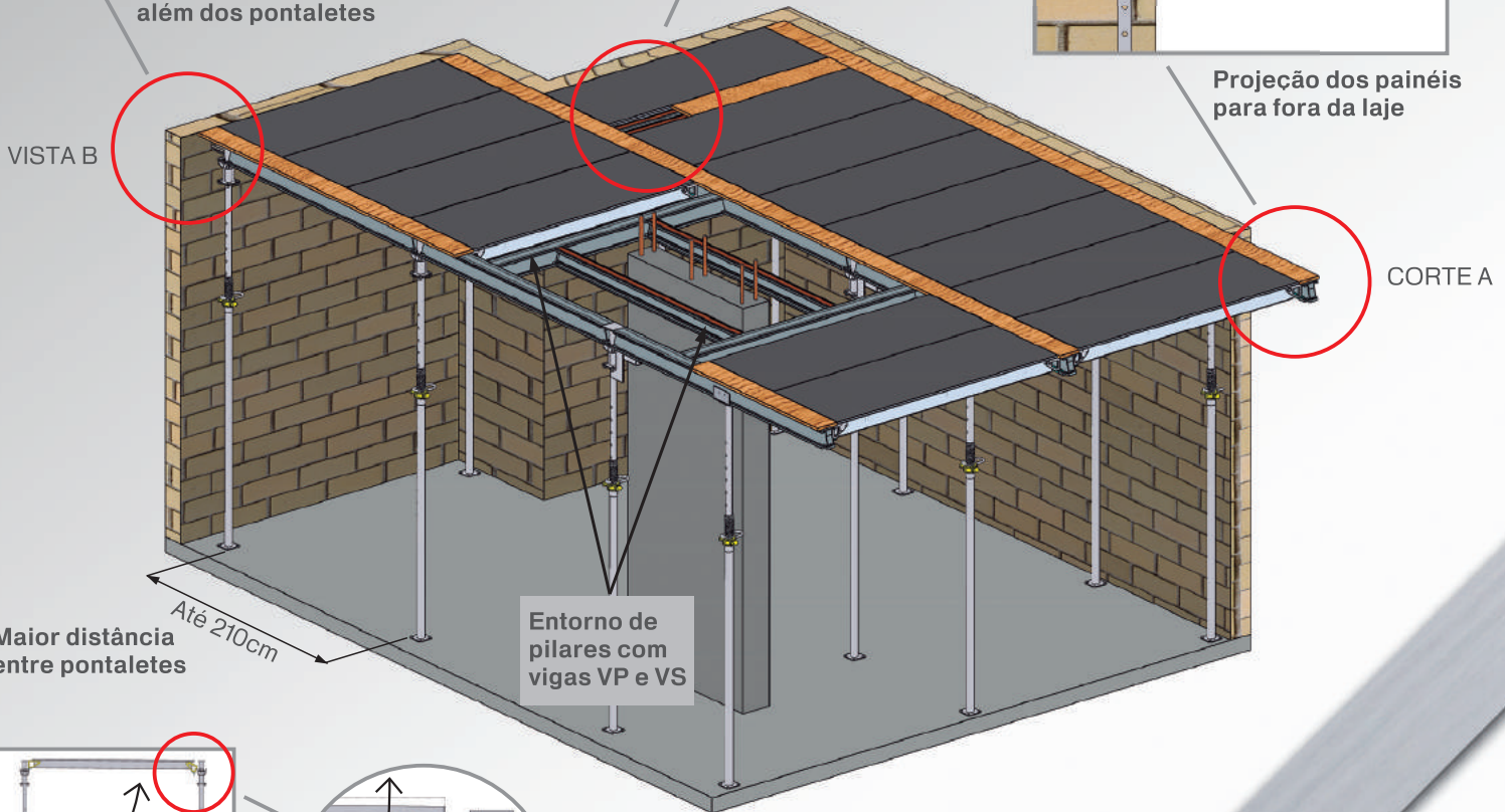
VISTA B Projeção dos painéis além dos pontaletes
