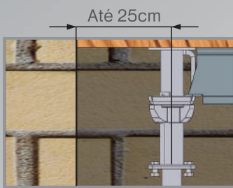
VISTA B Projeção dos painéis além dos pontaletes
